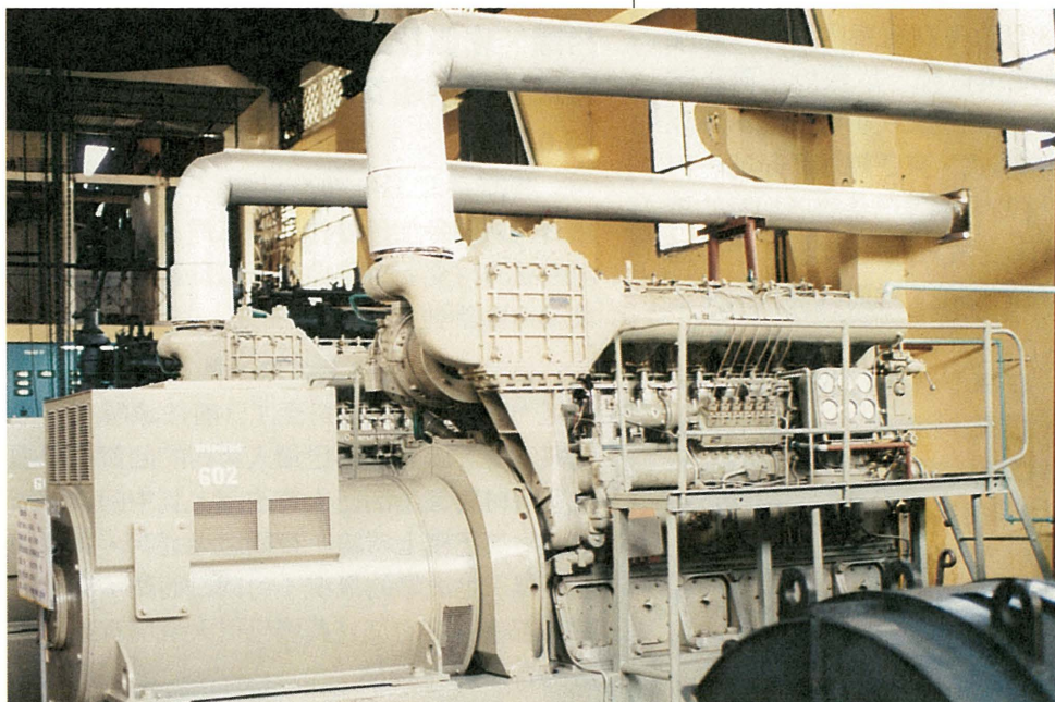
▲為協助柬埔寨人民自立，慈濟捐贈馬德旺省電廠三台發電機，接替即將報廢的老式機器。
